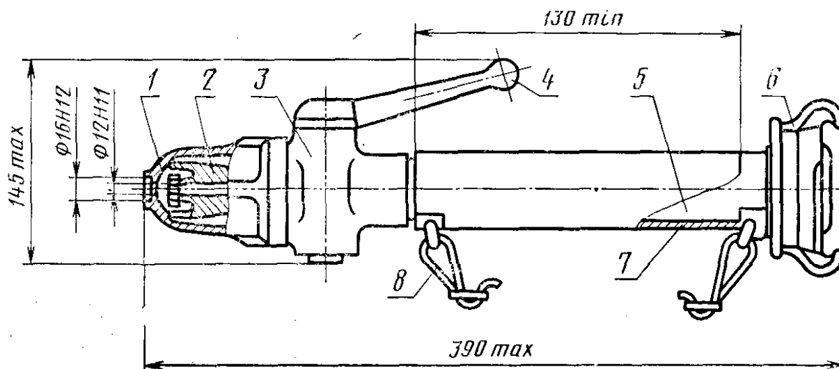
Чертеж. Основные параметры и размеры ствола
